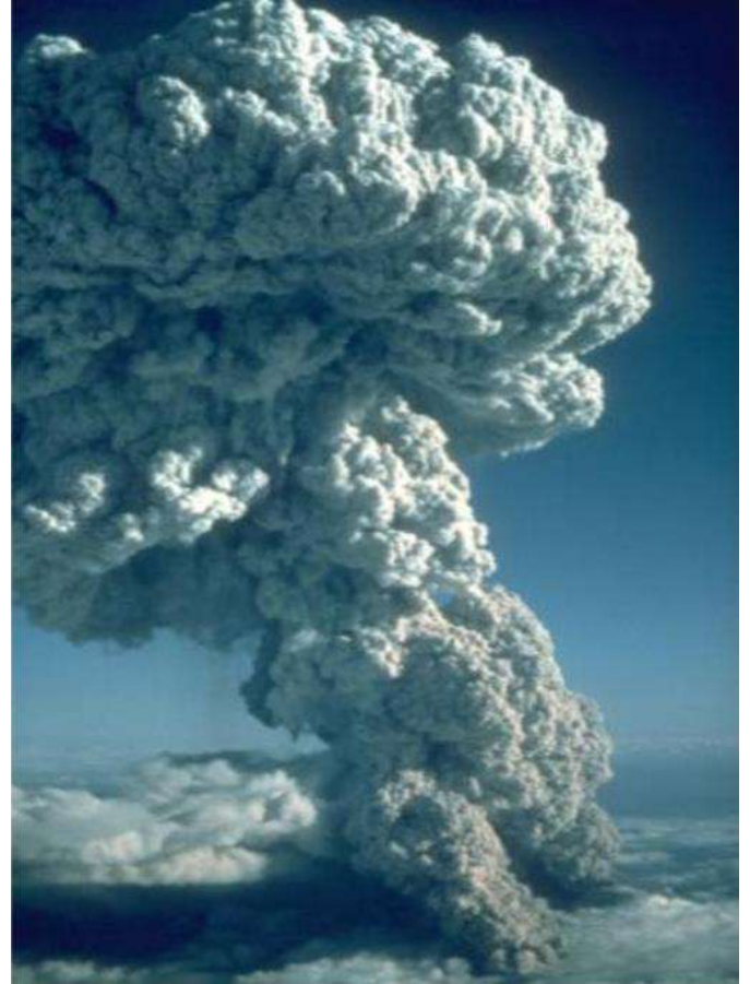
Eruption explosive du mont St. Helens le 22 juillet 1980, qui a produit une colonne d'éruption plinienne qui s'est élevée à 16 km au-dessus du volcan.
